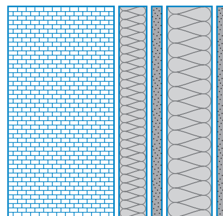
zdivo izolant vnější souvrství izolant nový vnější souvrství nové
