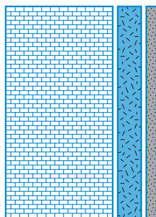
zdivo jádrová omítky vnější souvrství
