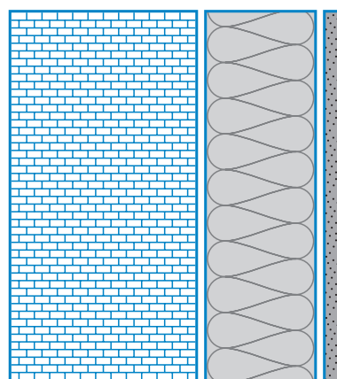
zdivo izolant vnější souvrství
